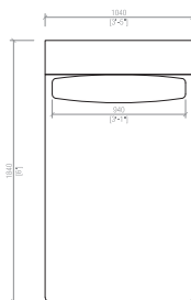
Chaise longue senza bracciolo Chaise longue without armrest cm 104x184 in 41"x72"4/9
