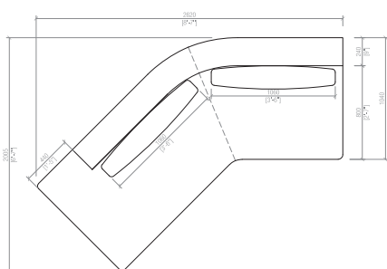
Elemento ad angolo B (dx/sx) Corner element B (L/R) cm 262x200 in 103"1/7x78"3/4
