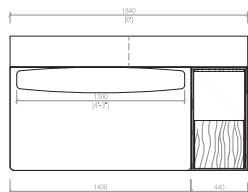
Centrale con tavolino integrato Central with integrated table cm 184x104 in 72"4/9x41"
