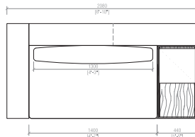
Laterale DX/SX con tavolino integrato Side R/L with integrated table cm 208x104 in 81"8/9x41"
