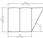
Elemento seduta angolo Corner seat element cm 120x82 in 47"1/4x32"2/7
