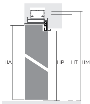
con traverso with header
